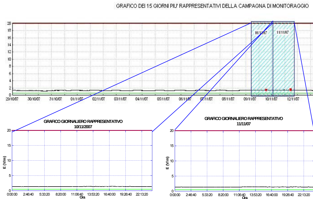
Figura 9: Grafico giornaliero rappresentativo (esempio)
