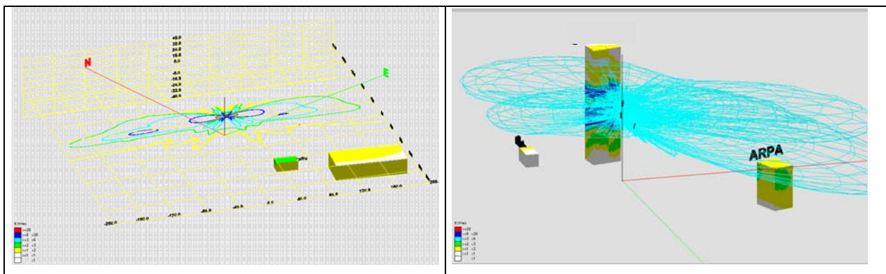
Simulazioni in 3D del Campo Elettrico generato da una SRB (al suolo ed in quota)
