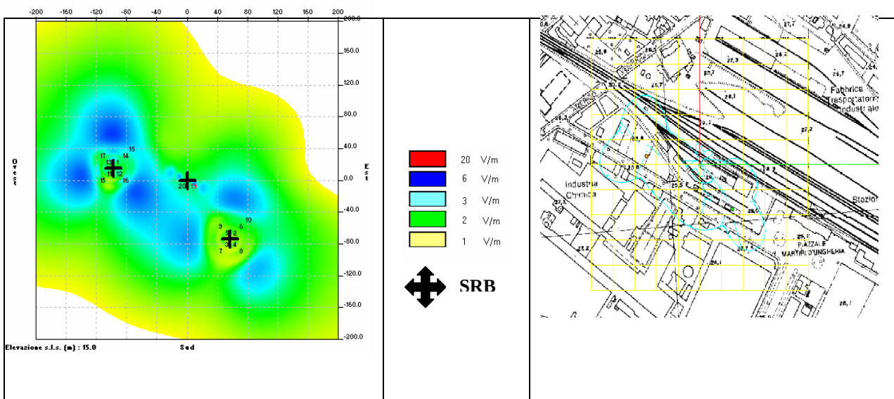
Mapa orizzontale del campo elettrico generato da più SRB; a sinistra con colori sfumati, a destra la stessa con isolinee di campo E riportate su cartografia CTR 1:5000
