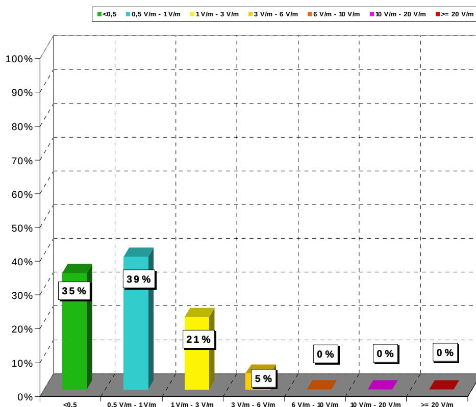
Figura 11: Distribuzione delle misure brevi
