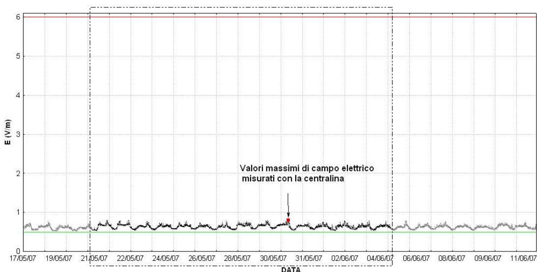
Figura 7: Grafico della campagna di monitoraggio
